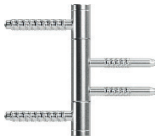
trojdielne pánty k zár. PORTA System - technický rozostup
