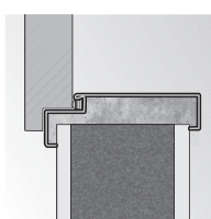
montáž bez dodatočných kotviacich elementov
