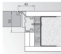
opačná polodrážka (otváranie dovnútra)
