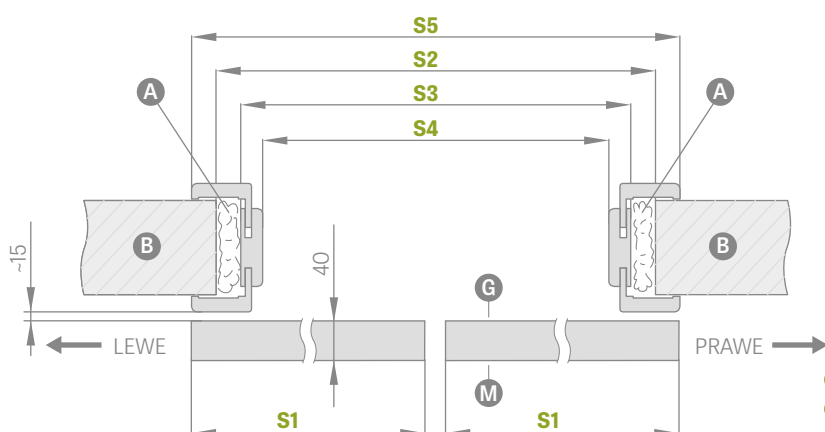
SP2N (verzia averz)
