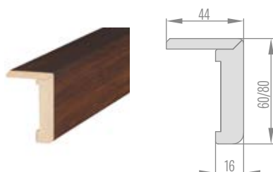
ŠTANDARDNÝ UHOLNÍK K REGULOVANEJ ZÁRUBŇI
