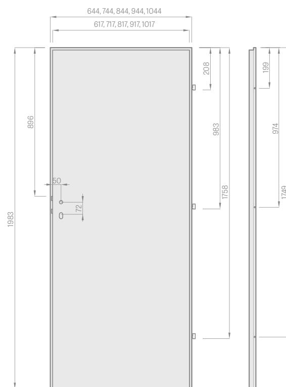
krídlo s polodrážkou
