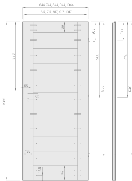
krídlo s polodrážkou
