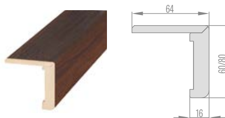
UHOLNÍK S PREDĹŽENÝM PEROM K REGULOVANEJ ZÁRUBŇI
